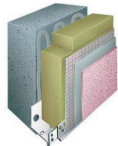
WDVS weber.therm A200 mit pas.top
